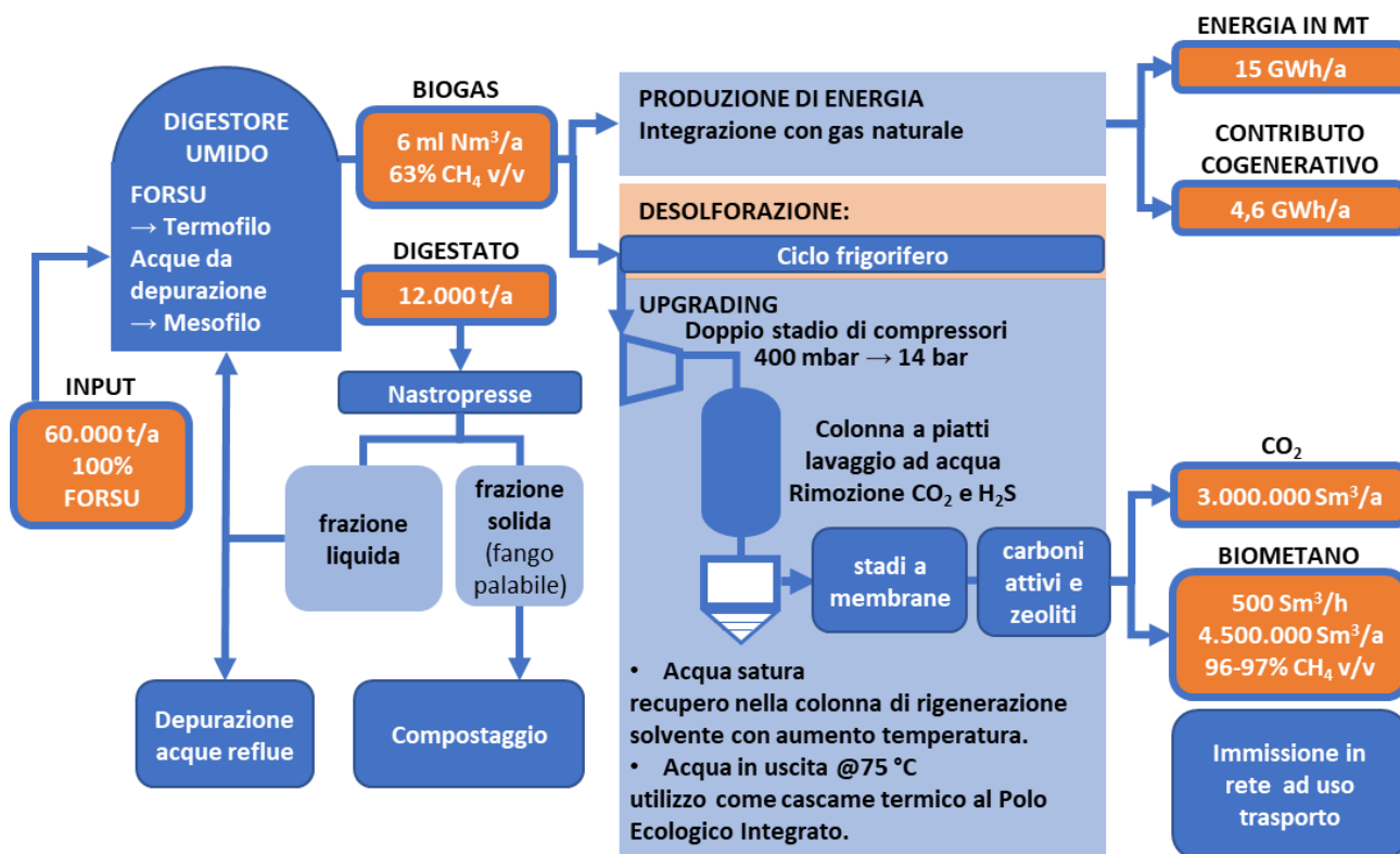
Figura 18 Schema dell'impianto di Acea Pinerolese
