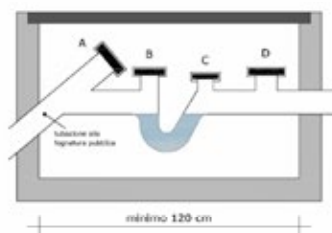
CAMERETTA DI ISPEZIONE TIPO BRAGA-SIFONE-ISPEZIONE (BSI)
