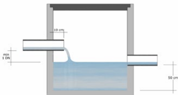
POZZETTO DI CAMPIONAMENTO
