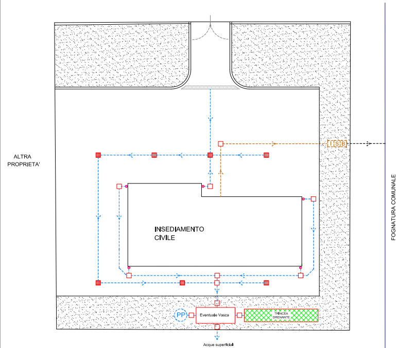
SCHEMA TIPO DI FOGNATURA PER INSEDIAMENTO CIVILE
