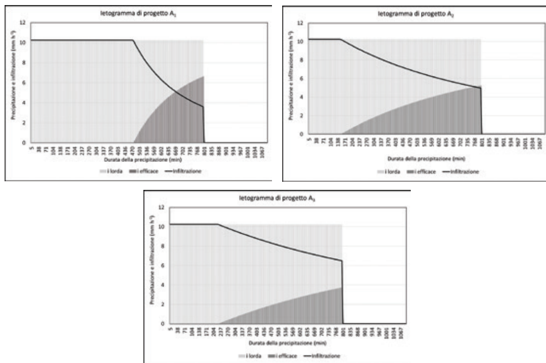
Figura 10. Pioggia totale, efficace e tasso d'infiltrazione delle tre superfici A1 (a), A2 (b) e A3 (c) nel caso di invaso addizionale pari a 41 mm e durata critica della precipitazione
