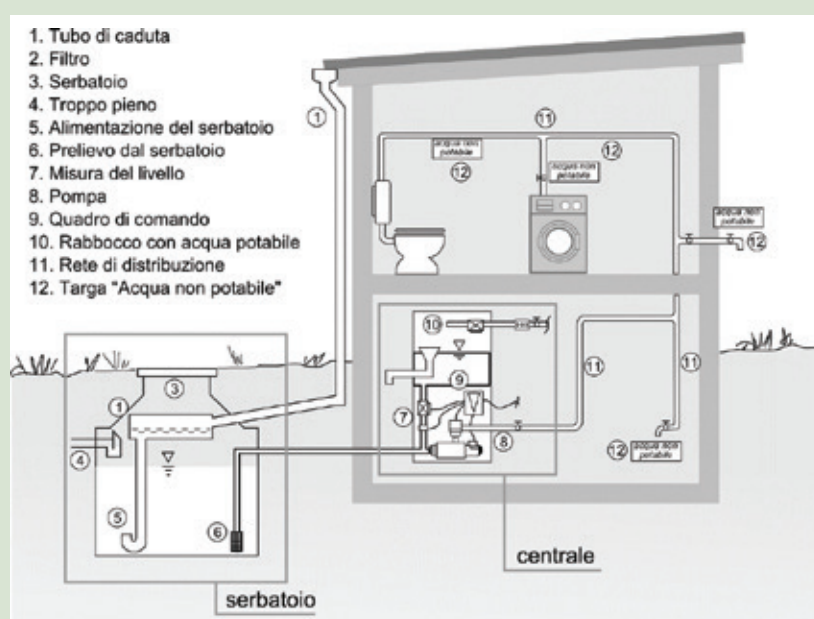
Figura 28. Schema d'impianto per molteplici usi domestici dell'acqua pluviale (Land Assia) (Tratta da: Di Fidio e Bischetti 2012).
