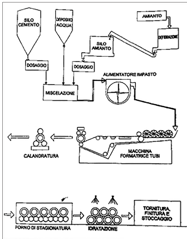
Figura 1 - Esempio di processo di lavorazione del cemento amianto (Progetto di bonifica amianto Sito da bonificare di interesse nazionale di Broni)
