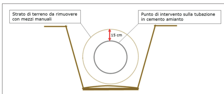
Figura 13 - Messa a giorno della tubazione idrica in cemento amianto.
